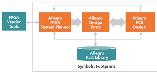
図 4: 既存ライブラリのシンボルやフットプリントが利用可能
